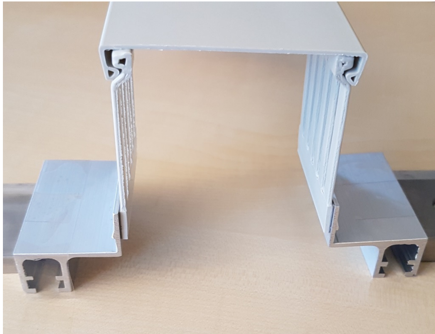
Example of use wiring profile with cover Anwendungsbeispiel Verdrahtungskämme mit Deckel
