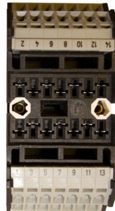
Sockel V29 AV mit Kodierung
