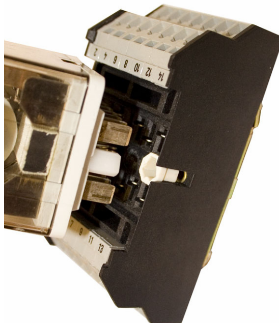
Anwendungsbeispiel für einen Sockel kodiert mit einem Relais kodiert.
