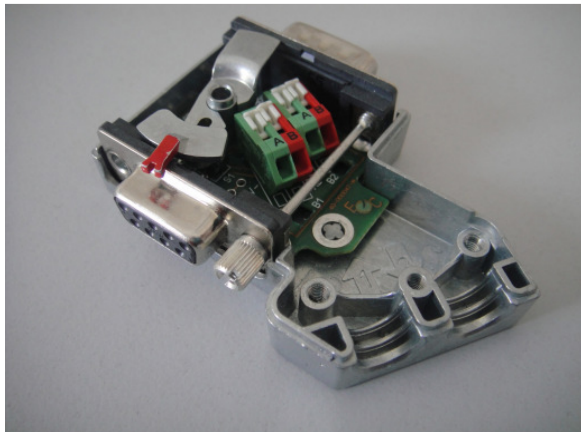
Sub-D (2 Kabeleingänge) mit Platine
