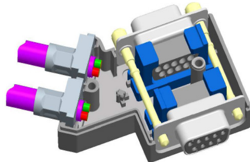
Sub-D (2 Kabeleingänge) mit Crimpflansch
